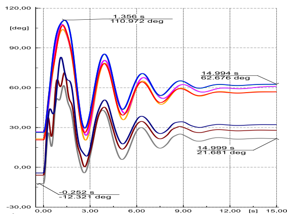
Fig. 6. Ángulos de rotor unidades sistema Sur.
