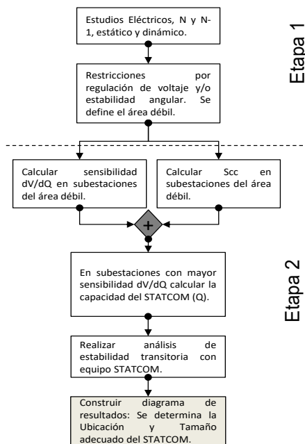
Fig. 2. Metodología para la ubicación y tamaño adecuado del STATCOM.
