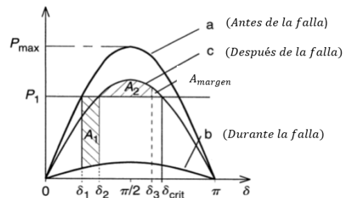
Fig. 1. Criterio de igualdad de áreas [13].
