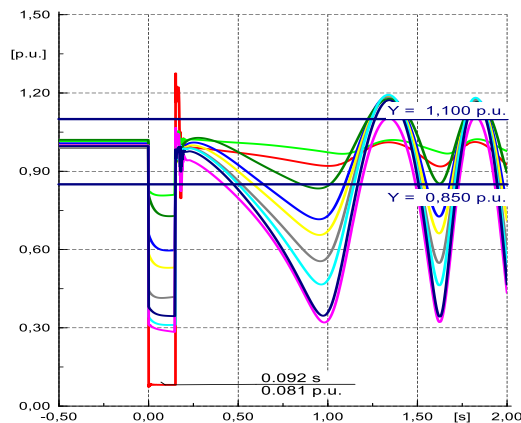
Fig. 5. Voltajes sistema Sur.
