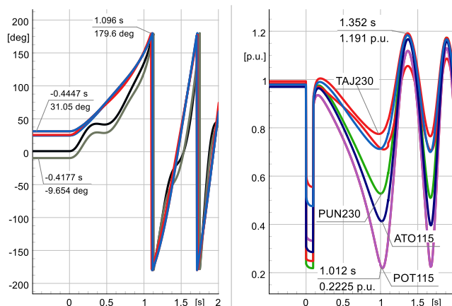
Fig. 4. Ángulos de rotor y voltajes sistema Sur.
