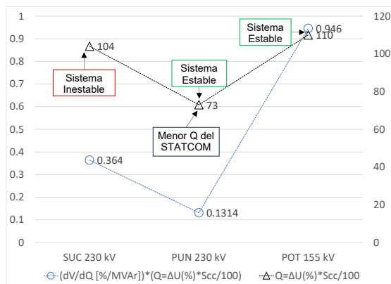
Fig. 9. Eje vertical derecho para Q (MVar) y eje izquierdo para \Delta U_a(\%) .
