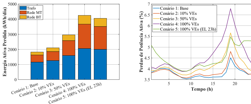
Fig. 9. Decomposição da energia ativa diária dissipada e evolução temporal percentual das perdas.
