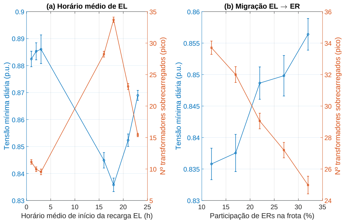
Fig. 12. Análise de sensibilidade da rede elétrica no Cenário 4.
