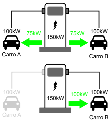
Fig. 1. Representação do fator de balanço de potência em eletropostos rápidos.
