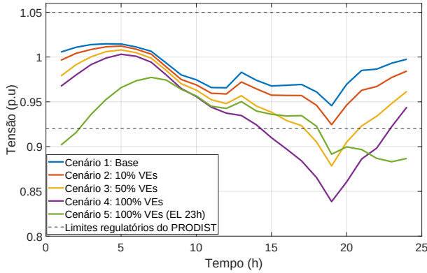
Fig. 6. Perfil médio diário do valor mínimo de tensão nas barras de baixa tensão.
