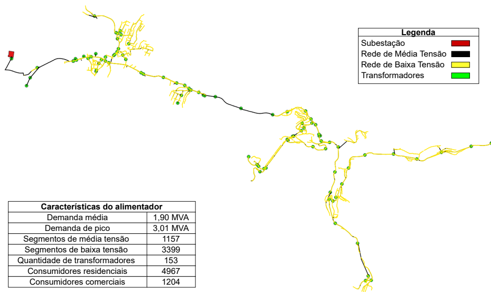
Fig. 5. Alimentador escolhido para o estudo de caso.
