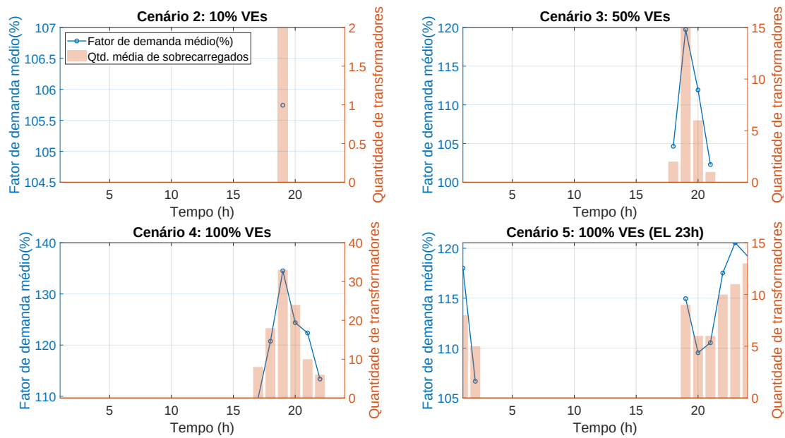
Fig. 8. Análise temporal da sobrecarga de transformadores baseada no fator de demanda médio obtido via simulação de Monte Carlo.
