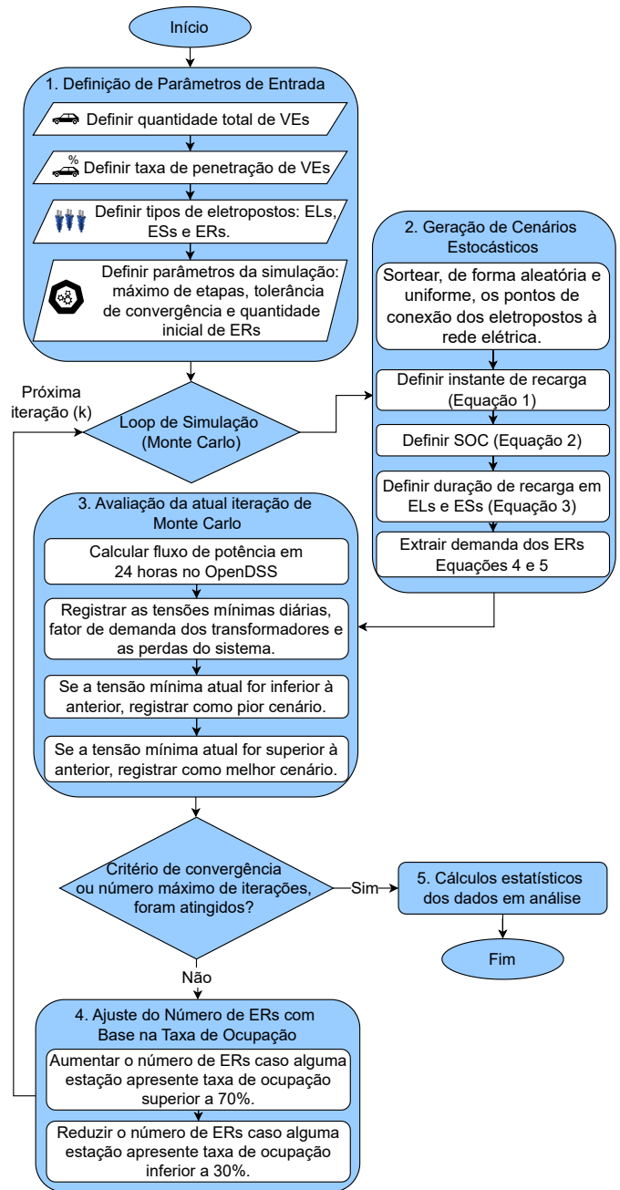
Fig. 4. Método da simulação de Monte Carlo para inserção de eletropostos na rede de distribuição.
