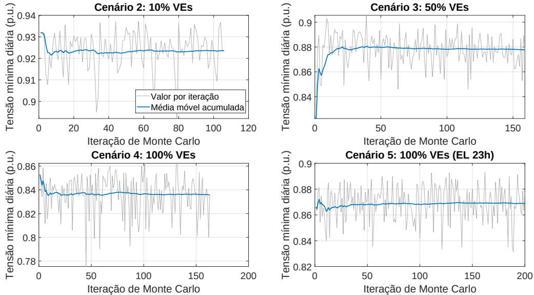
Fig. 7. Convergência de Monte Carlo e dispersão da tensão mínima diária por cenário.
