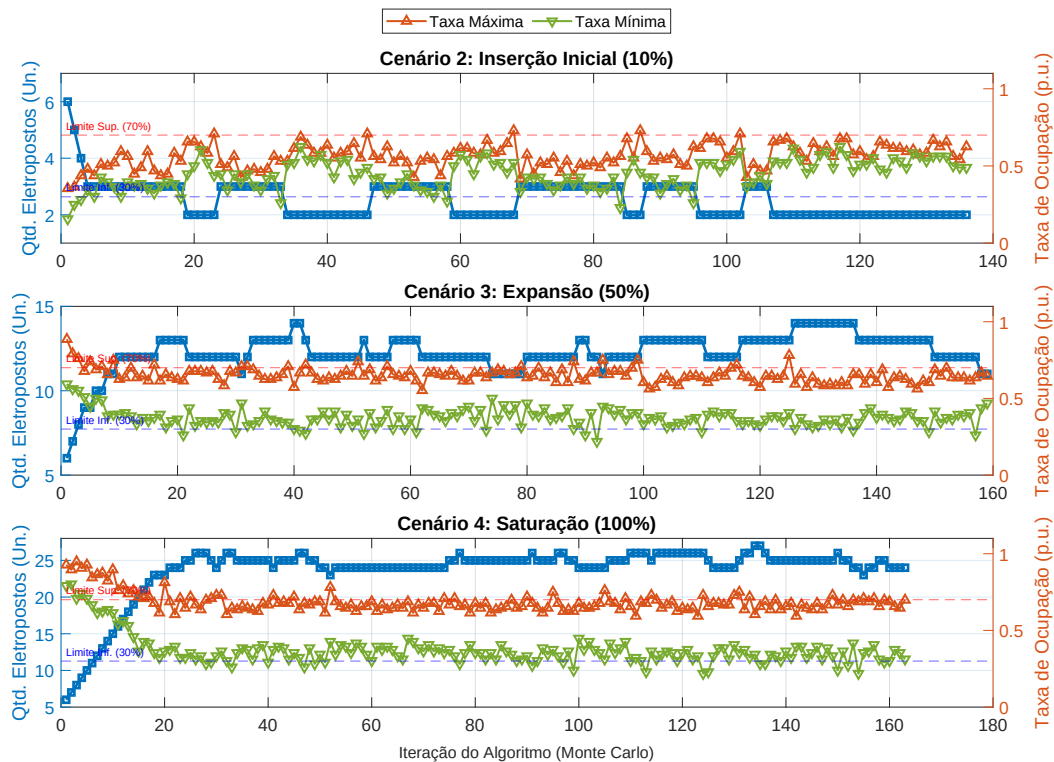
Fig. 10. Quantidade de eletropostos rápidos de acordo com a taxa de ocupação no processo de Simulação de Monte Carlo.
