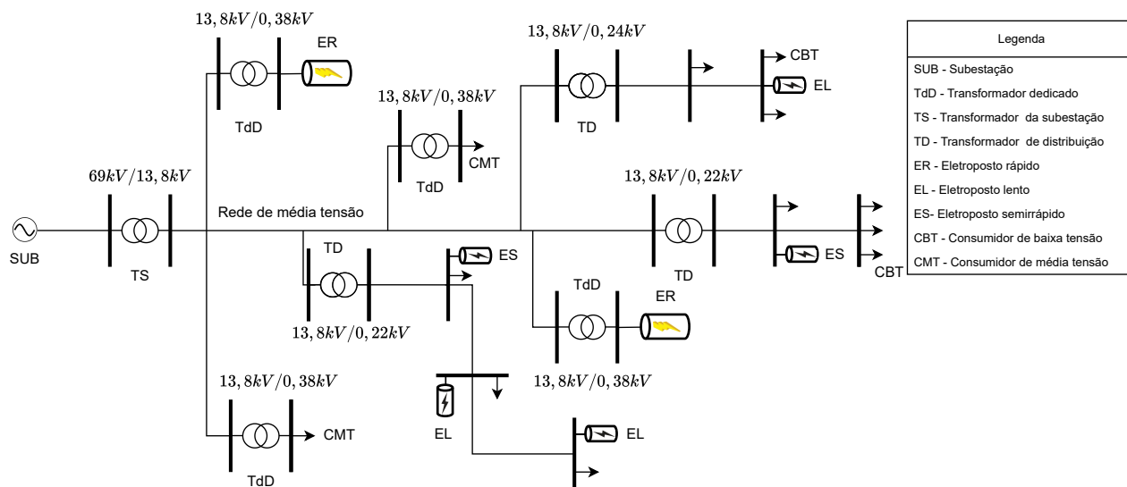
Fig. 2. Representação esquemática da rede modelada.
