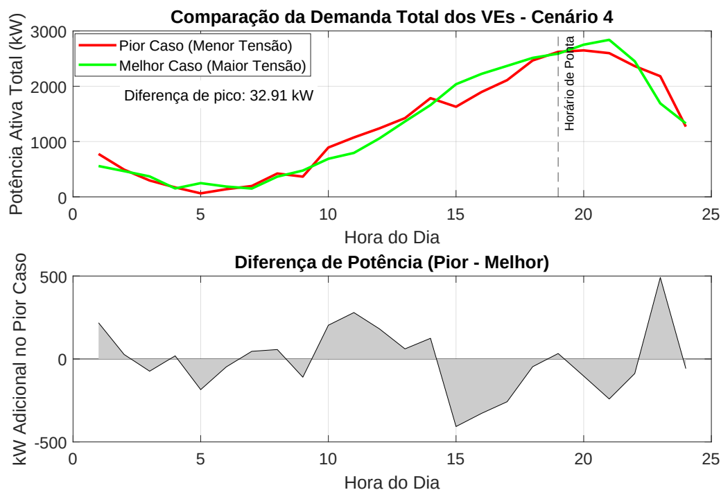
Fig. 11. Comparação da demanda total dos VEs - Cenário 4
