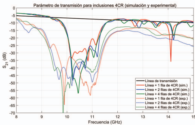
Fig. 8. Parámetro de transmisión para inclusiones de tipo 4CR (simulación -líneas continuas- y experimental -líneas de puntos-).
