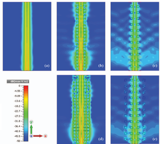
Fig. 9. Amplitud del campo eléctrico en la superficie del sustrato dieléctrico para una frecuencia de 9.5 GHz, fuera de la banda prohibida: (a) línea de transmisión, (b) línea de transmisión con una fila de mushrooms , (c) línea de transmisión con una fila de 4CR, (d) línea de transmisión con dos filas de mushrooms , (e) línea de transmisión con dos filas de 4CR. Todas las figuras con la misma escala.
