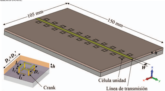
Fig. 3. Línea microstrip con una fila de celdas formadas por cuatro manivelas (4CR) a cada lado y detalle de la celda unidad de manivelas.
