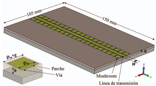
Fig. 2. Línea microstrip con una fila de mushrooms a cada lado y detalle del mushroom .
