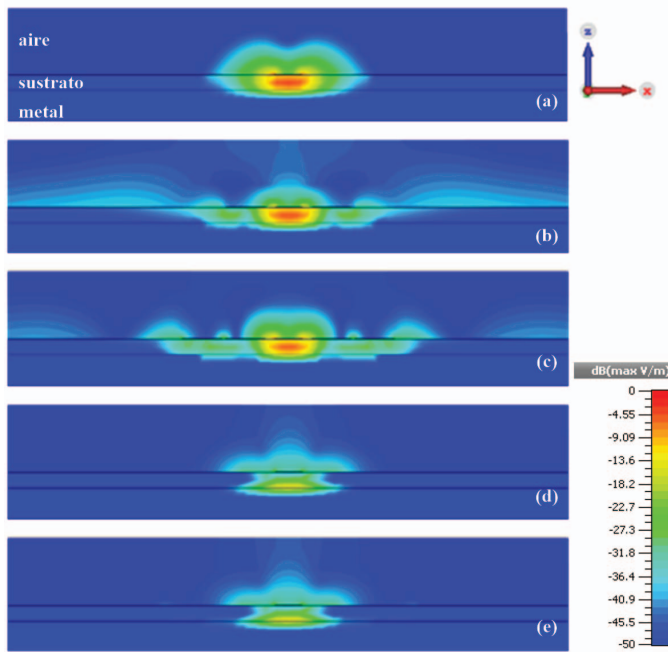
Fig. 11. Magnitud del campo eléctrico en el plano XZ ( y = 30 mm): (a) línea de transmisión a 11.25 GHz, (b) línea con una fila de mushrooms a 11.5 GHz, (c) línea con dos filas de mushroom a 10.82 GHz, (d) línea con una fila de 4CR a 10.9 GHz, y (e) línea con dos filas de 4CR a 10.9 GHz.
