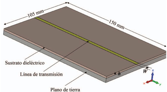
Fig. 1. Línea microstrip de impedancia característica 50 \Omega .
