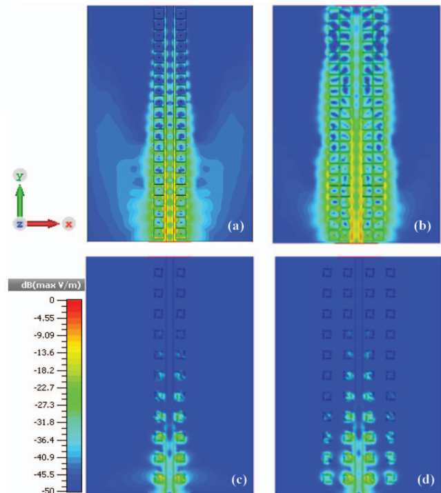
Fig. 10. Amplitud del campo eléctrico en la superficie del sustrato dieléctrico a diferentes frecuencias: (a) una fila de mushrooms (11.5 GHz), (b) dos filas de mushrooms (10.82 GHz), (c) una fila de 4CR (10.9 GHz), (d) dos filas de 4CR (10.9 GHz). Todas las figuras con la misma escala.
