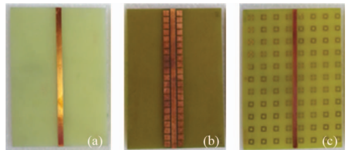
Fig. 4. Modelo implementado en sustrato FR-4: (a) línea de transmisión sin inclusiones, (b) línea de transmisión con inclusiones en forma de mushrooms y (c) línea de transmisión con inclusiones 4CR.
