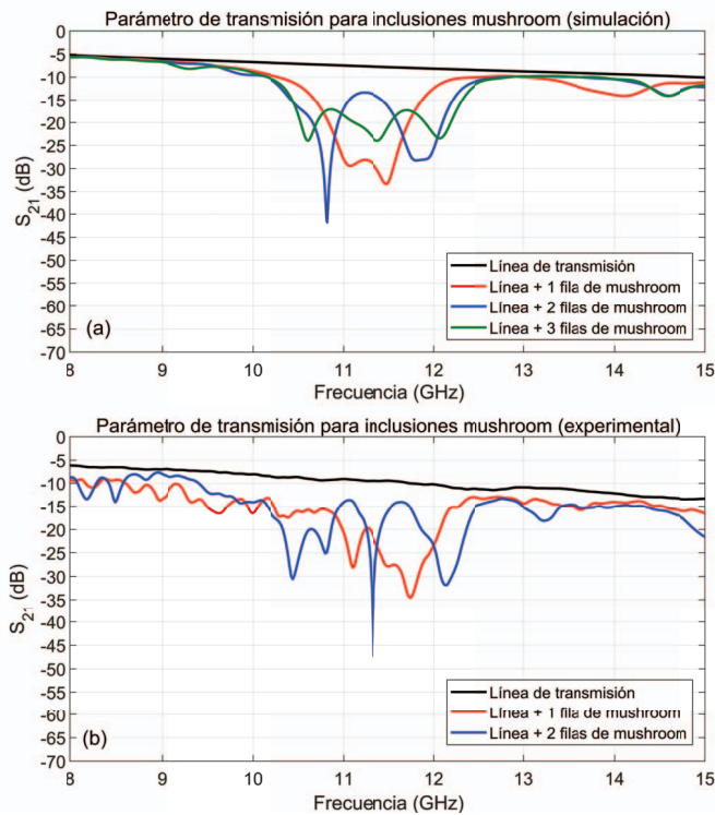
Fig. 5. (a) Simulación numérica. Parámetro de transmisión de la línea microstrip (negro), línea microstrip con una fila de mushrooms (rojo), con dos filas de mushrooms (azul) y con tres filas de mushrooms (verde). (b) Medidas experimentales. Igual para una y dos filas de mushrooms .
