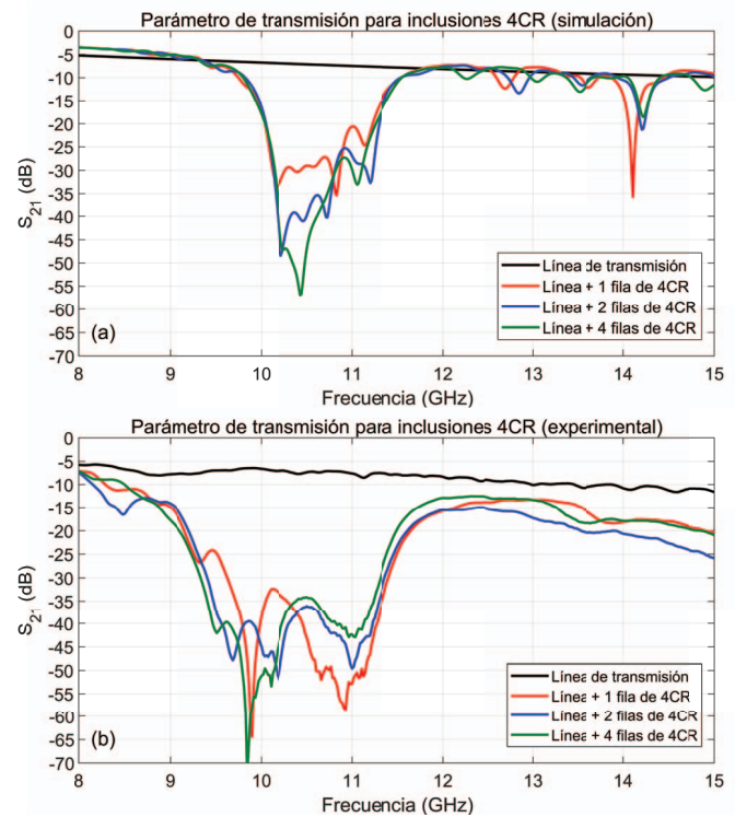
Fig. 6. (a) Simulación numérica. Parámetro de transmisión de la línea microstrip (negro), línea con una fila de inclusiones (rojo), con dos filas de inclusiones (azul) y con tres filas de inclusiones (verde). (b) Medidas experimentales. Igual para una y dos filas de inclusiones 4CR.
