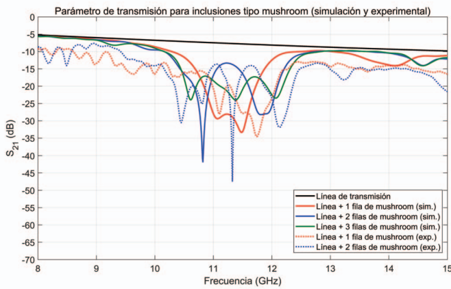
Fig. 7. Parámetro de transmisión para inclusiones de tipo mushroom (simulación -líneas continuas- y experimental -líneas de puntos-).
